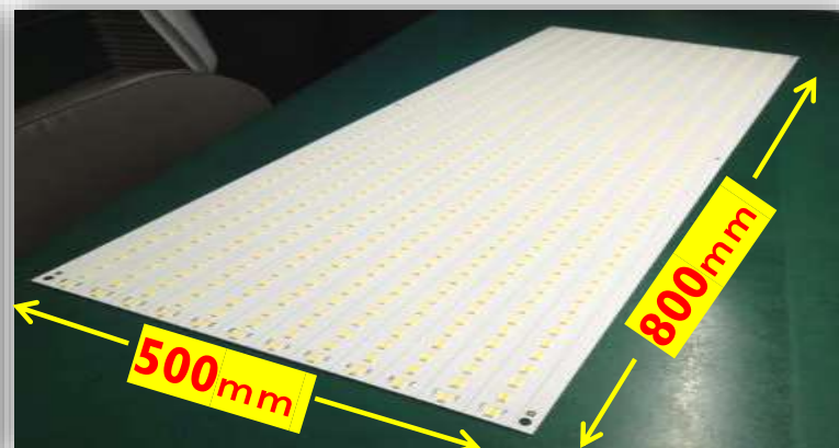
LED基板 最大 (800mm x 500mm)
