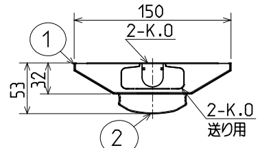
側面詳細図
