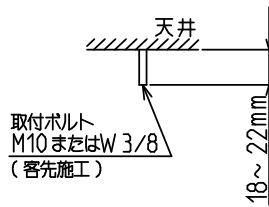
器具取付ボルト長さ
