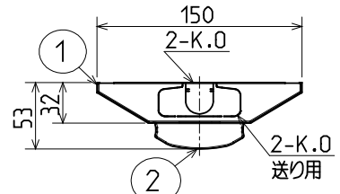
側面詳細図
