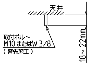
器具取付ボルト長さ
