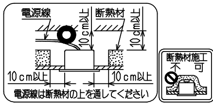
断熱施工天井への施工方法
