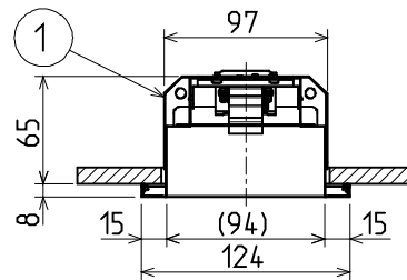
側面詳細図
