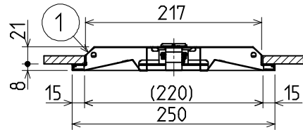
断面詳細図
