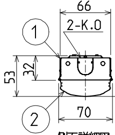
側面詳細図
