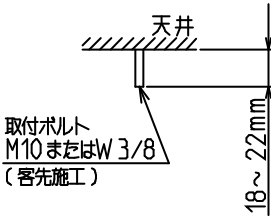
器具取付ボルト長さ
