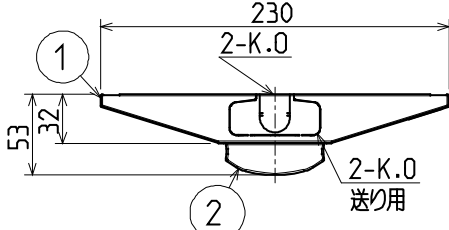
側面詳細図
